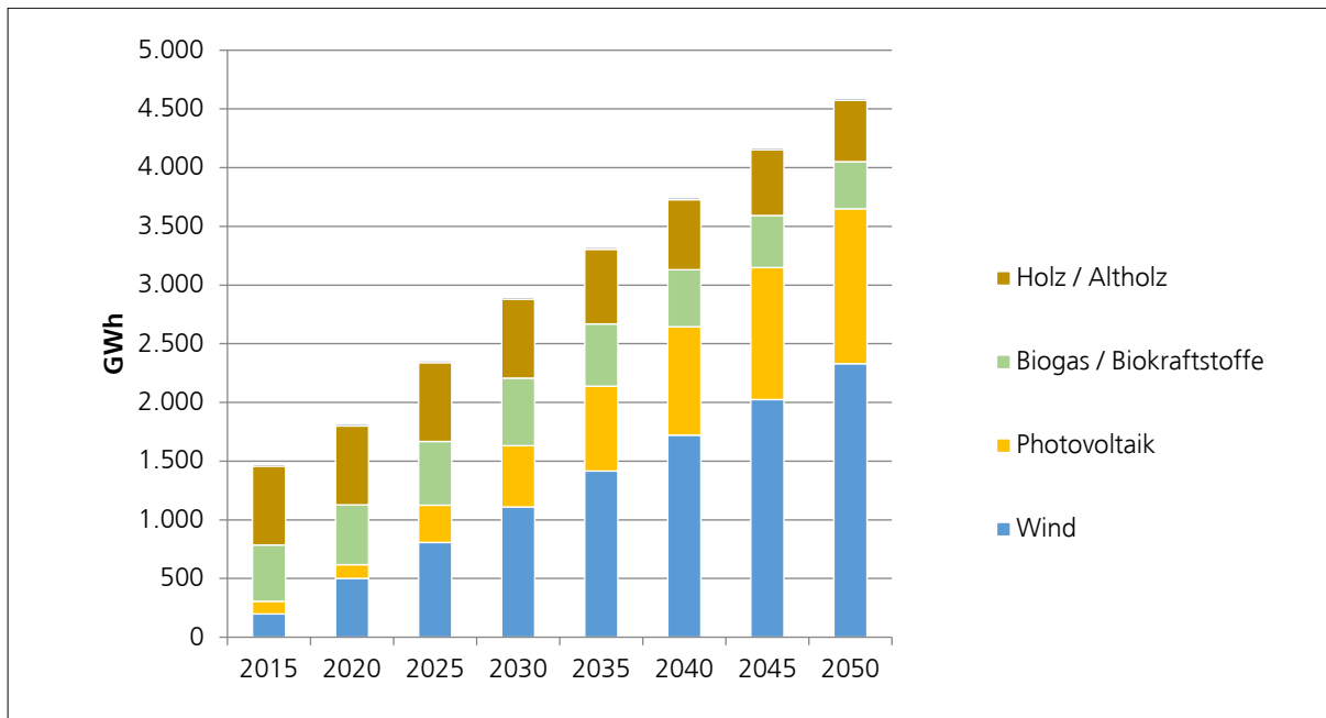
Abbildung 40: Entwicklung der Nutzung erneuerbarer Energien im Szenario Klimaneutralität bis 2050 in der Region Weserbergland
