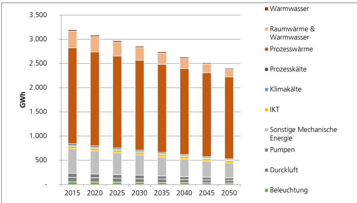
Abbildung 24: Energieeinsparpotenzial (Strom und Brennstoffe) bis 2050 im Sektor Industrie in der Region Weserbergland
