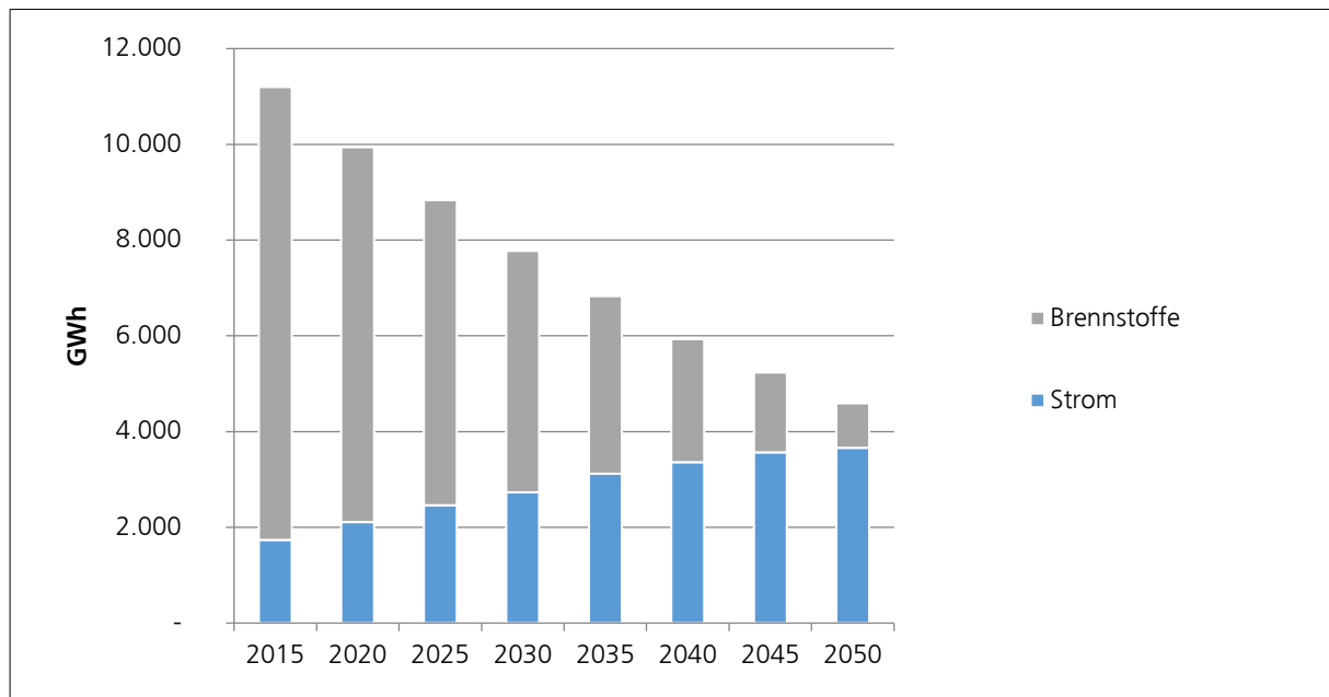
Abbildung 39: Entwicklung der Elektrifizierung der Energieversorgung im Szenario Klimaneutralität bis 2050 in der Region Weserbergland
