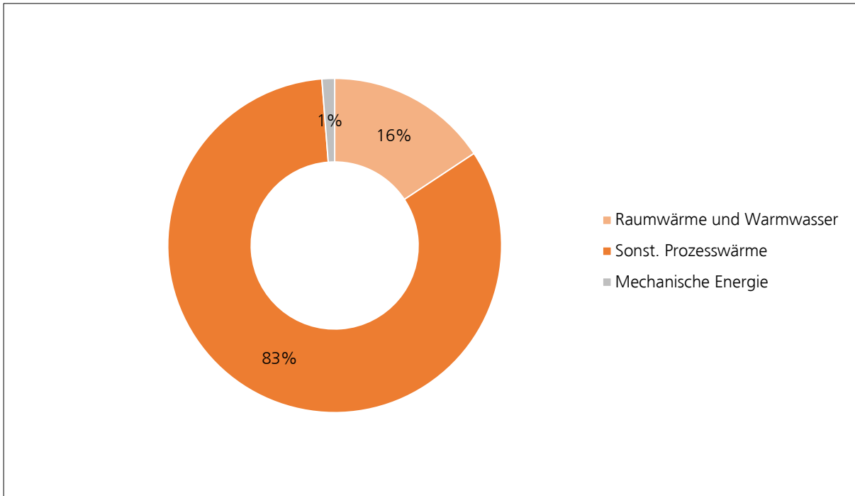
Abbildung 23: Brennstoffverbrauch im Unter-Sektor Industrie nach Energieanwendungen ohne Hot Spots 2015 in der Region Weserbergland
