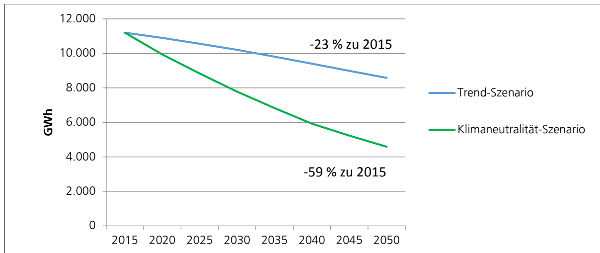
Abbildung 42: Entwicklung des Endenergieverbrauchs im Trend-Szenario und im Szenario Klimaneutralität bis 2050 in der Region Weserbergland
